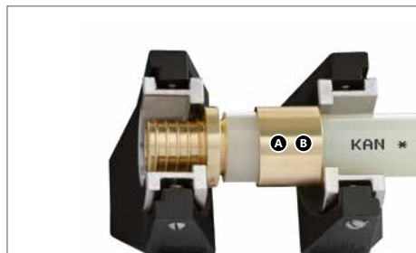
Montaż łączników \varnothing 12 \times 2 , \varnothing 14 \times 2 , \varnothing 18 \times 2 , \varnothing 18 \times 2,5
