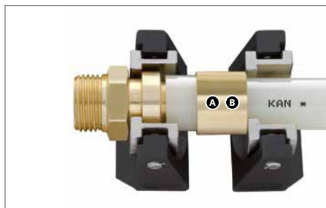
Montaż złączek z GZ i GW Ø12x2, Ø14x2, Ø18x2, Ø18x2,5
