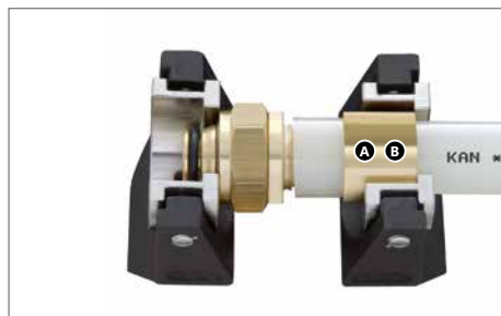
Montaż śrubunka z pierścieniem nasuwanym
