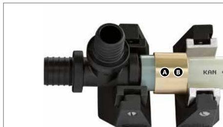
Montaż kolan i trójników PPSU \varnothing 25 \times 3,5
