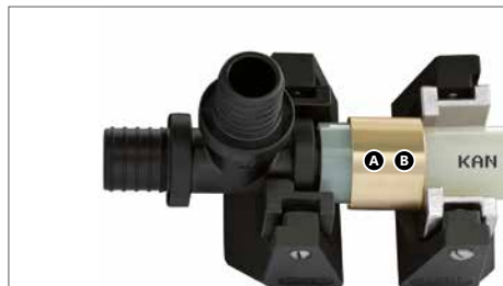
Montaż kolan i trójników PPSU \varnothing 12 \times 2 , \varnothing 14 \times 2 , \varnothing 18 \times 2 , \varnothing 18 \times 2,5
