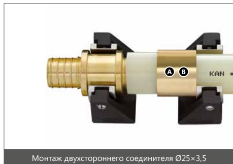
Монтаж двухстороннего соединителя Ø25×3,5
