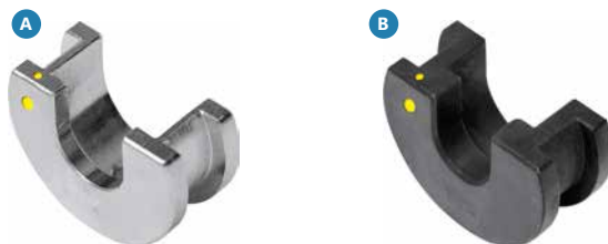
Rys. 7 Wkładki proste do praski (a - nikielowany, b - czarny)
