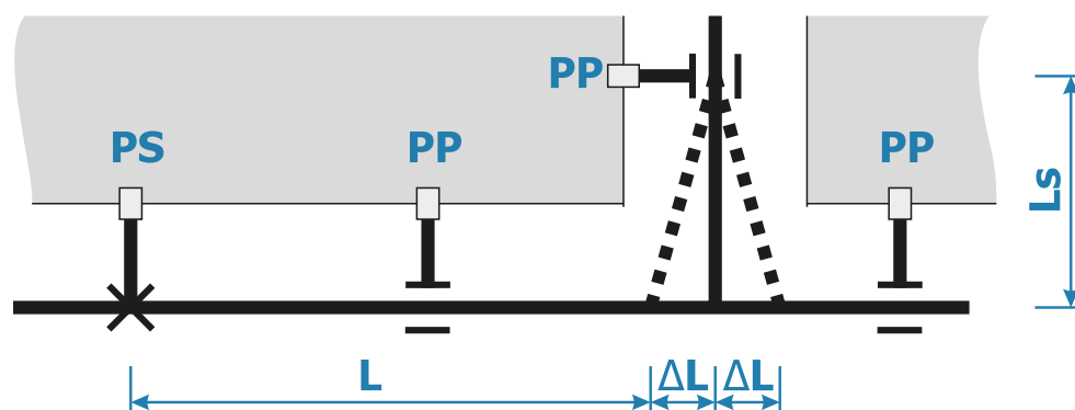
Определение компенсационного плеча на ответвлении
