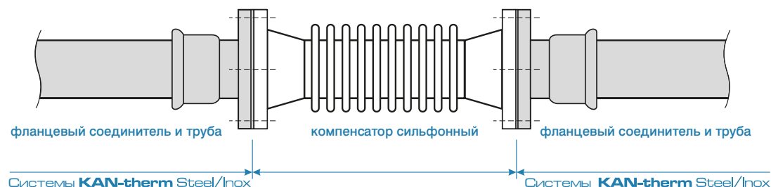
Компенсатор сифонный для стальных труб (пример)
