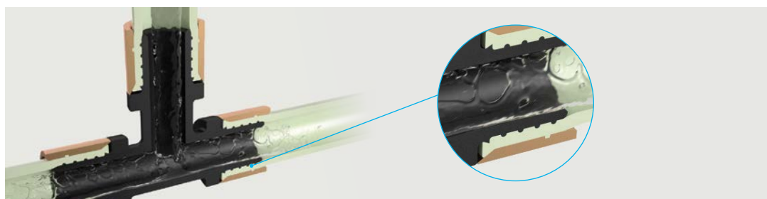
Соединение Push в разрезе
