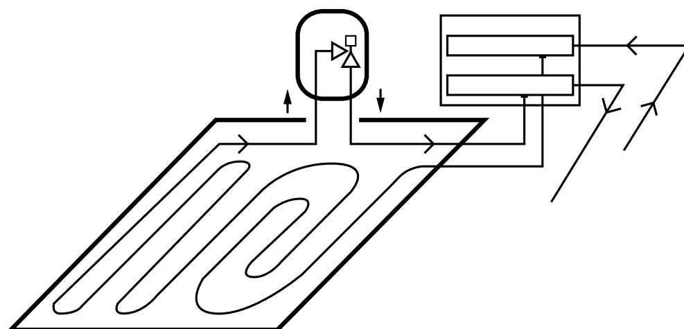
Рис. 72. Схема работы – комплект расположен на обратке.
