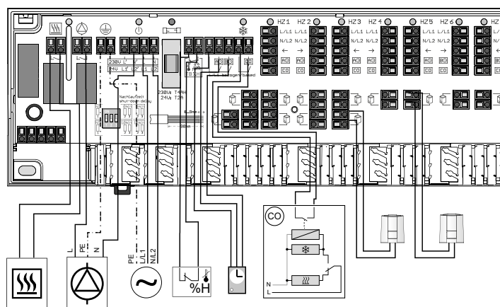
Рис. 67. Конфигурация клеммной колодки Basic+ 230В или 24В с насосным модулем
