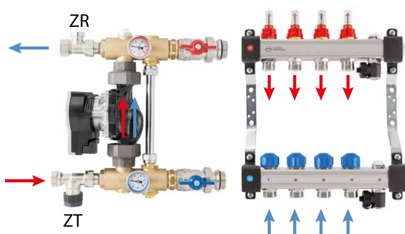
Рис. 53. Насосная группа 1346103000 с распределителем серии UFST – направления потоков воды
