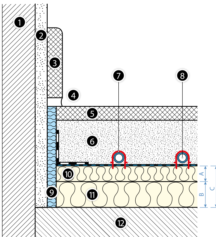
Рис. 22. Подпольный отопительный прибор с системной плитой KAN-therm Tacker и дополнительной изоляцией на перекрытии над неотапливаемым внутренним помещением, а также перекрытием контактирующим с наружным воздухом
