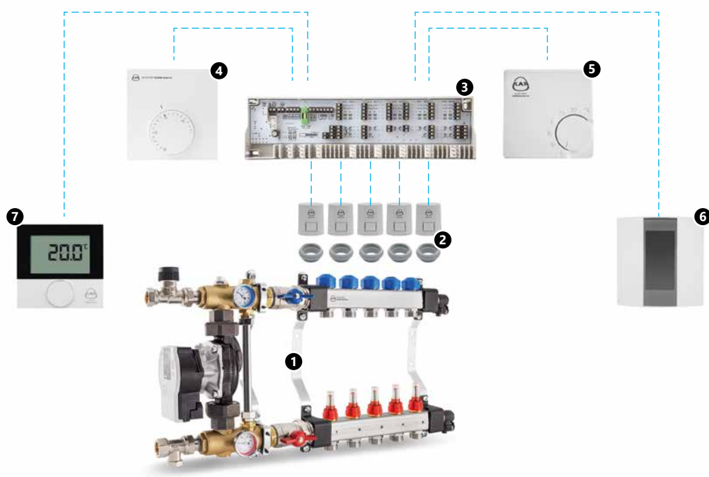
Рис. 55. Примерная конфигурация местной проводной автоматики KAN-therm в панельном отоплении
