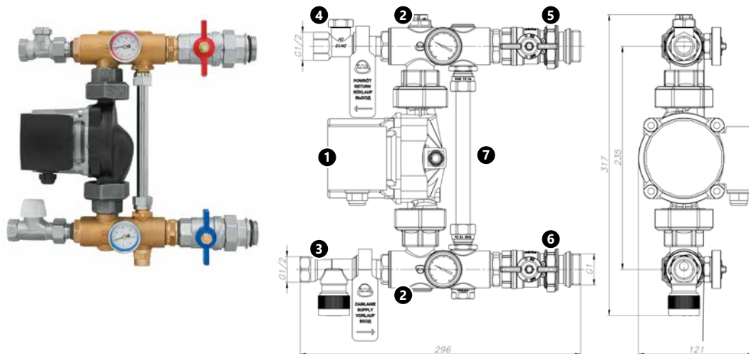
Рис. 48. Конструкция смесительного узла на базе насосной группы KAN-therm
