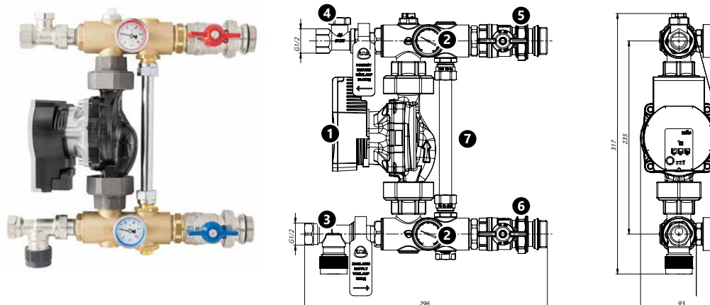
Рис. 49. Конструкция смесительного узла на базе насосной группы KAN-therm
