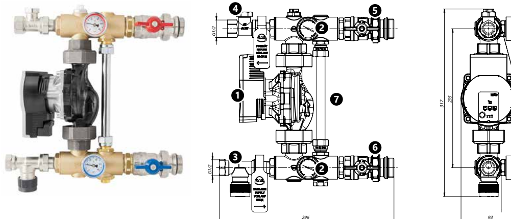
Рис. 50. Конструкция насосной группы KAN-therm с электронным насосом
