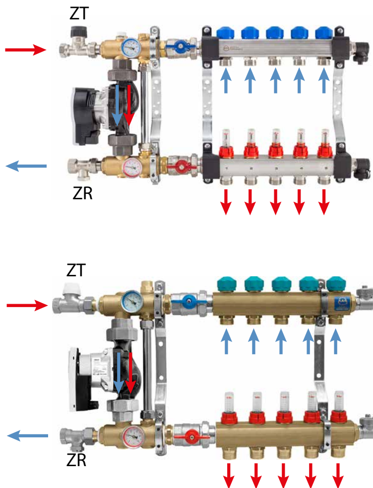
Рис. 52. Распределитель со смесительной системой серии USFP и 77E – направления потоков воды
