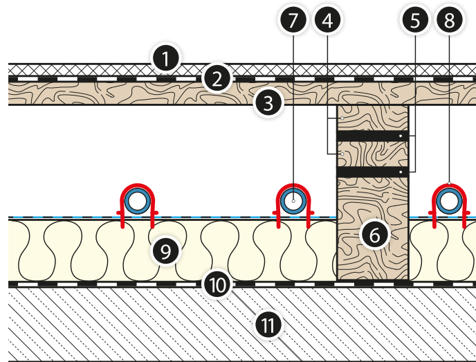
Рис. 31. Конструкция спортивного поверхностно-эластичного пола с системой подпольного отопления, выполненного из элементов системы KAN-therm Tacker.
