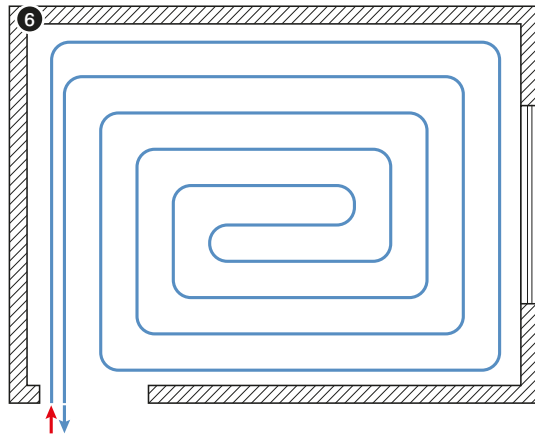
Рис. 6. Контур подпольного отопления/охлаждения в форме спирали (улитки).
